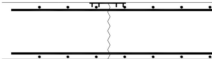
c) těsnící pásy venkovní
