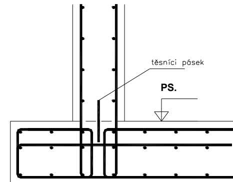
b) - upravená, těsnící pásek úpravená výztuž
