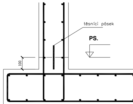
a) - upravená, těsnící pásek zvýšená spára
