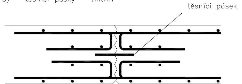
b) – těsnící pásy – vnitřní
