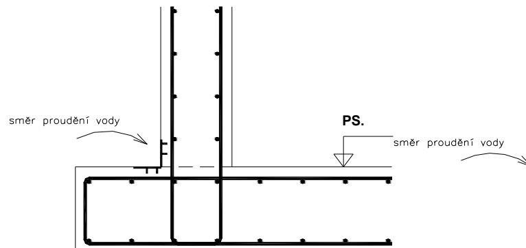
c) - rohový těsnící pás
