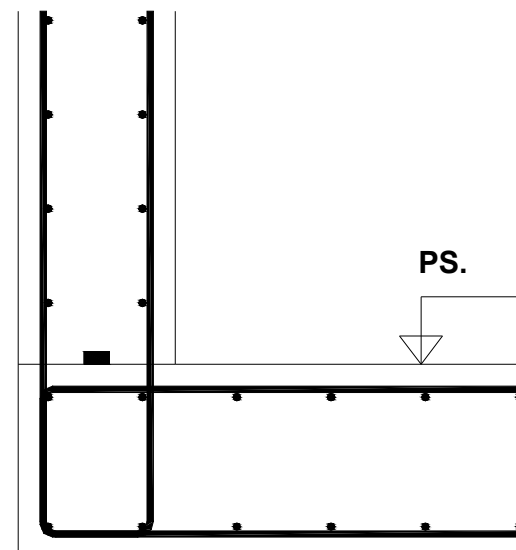
b) – bentonitové bobtnavé těsnící pásky
