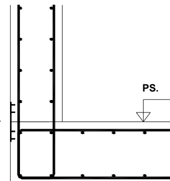
d) - venkovní těsnící pás
